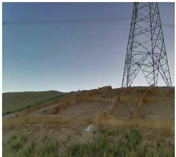
流坡草方格治理
